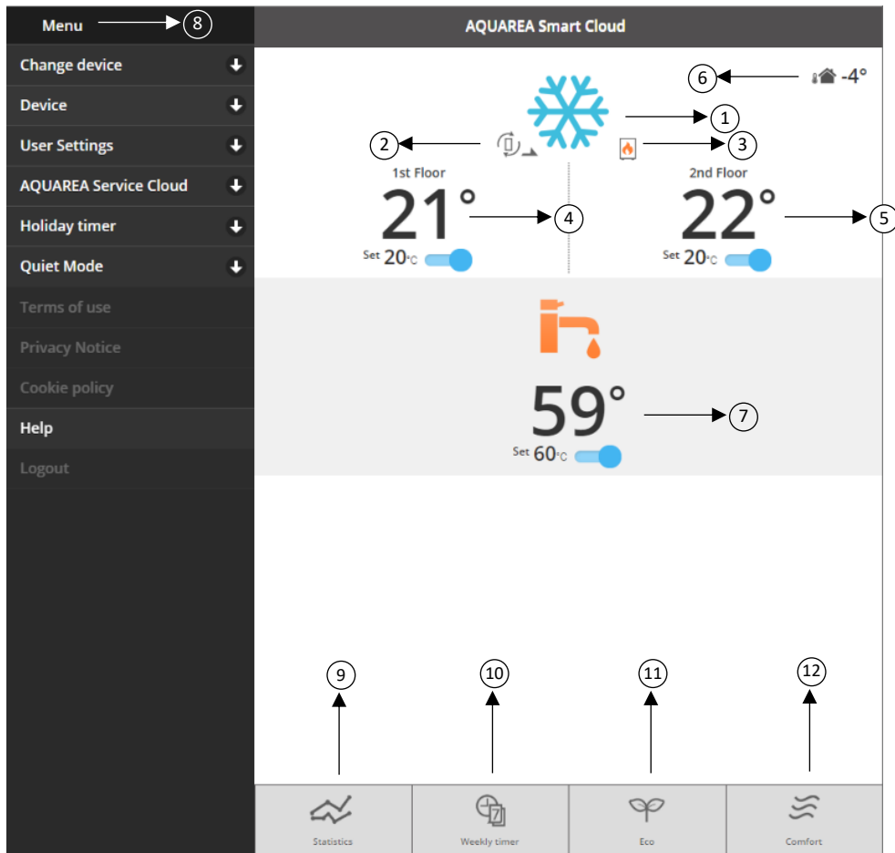
14 pav. Operacijos ekranas
