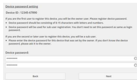
Εικόνα 13 - Ορισμός κωδικού πρόσβασης για αυτήν τη συσκευή - Βήμα 3
