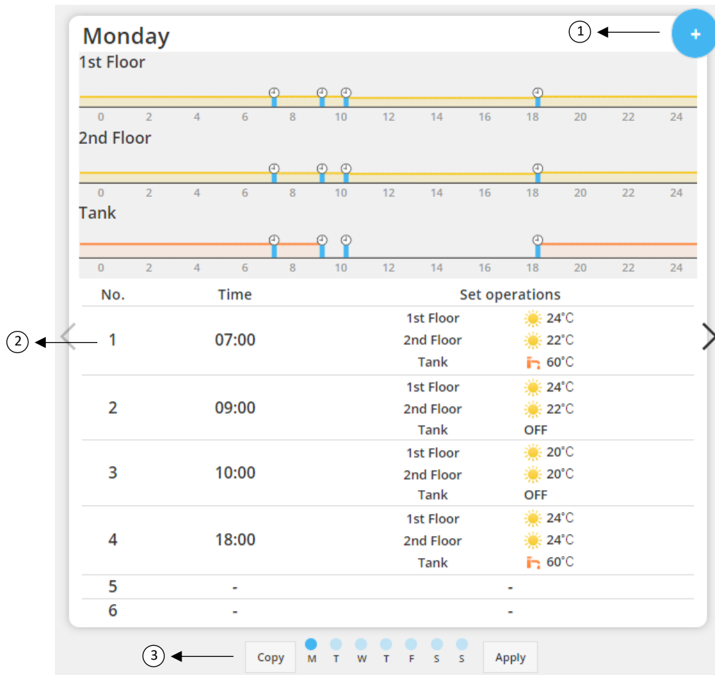
Εικόνα 20 – Ρύθμιση εβδομαδιαίου χρονοδιακόπτη
