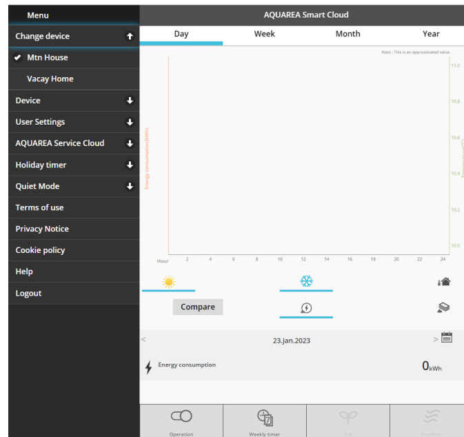
Εικόνα 27 - Αλλαγή συσκευής
