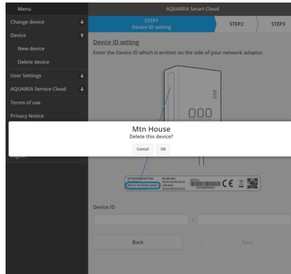
Εικόνα 28 - Διαγραφή συσκευής
