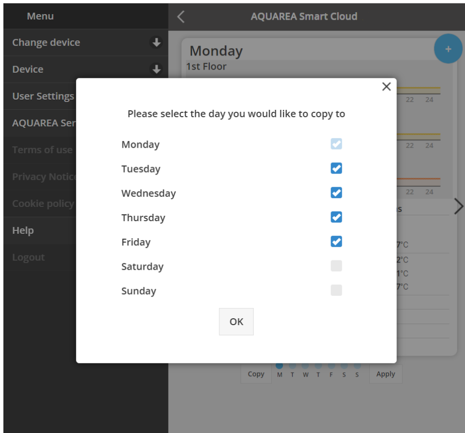
Εικόνα 21 - Μενού αντιγραφής
