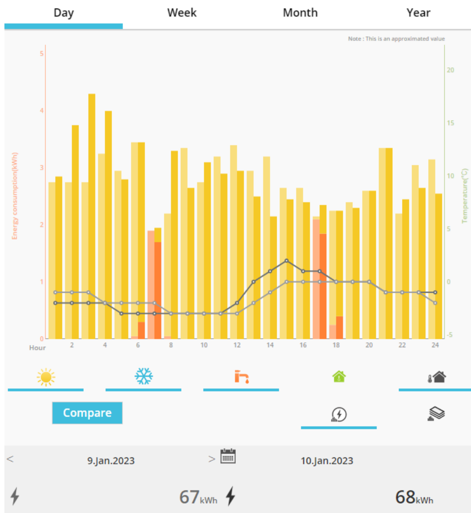
Εικόνα 18 - Γράφημα σύγκρισης
