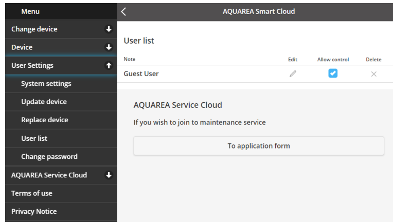
Εικόνα 32 - Λίστα χρηστών
